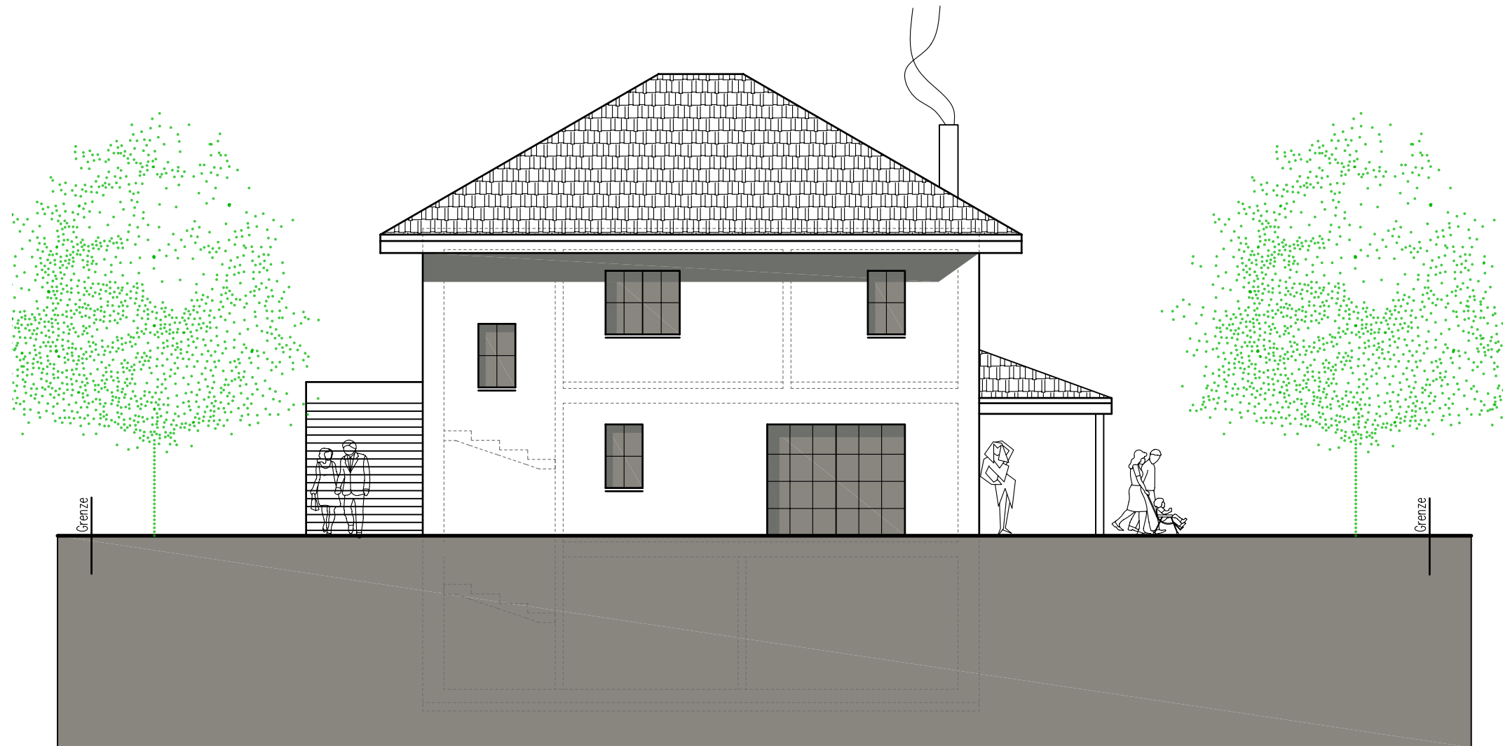
West-Fassade Mst. 1:100
